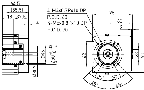
Motor Adaptor Flange F1
